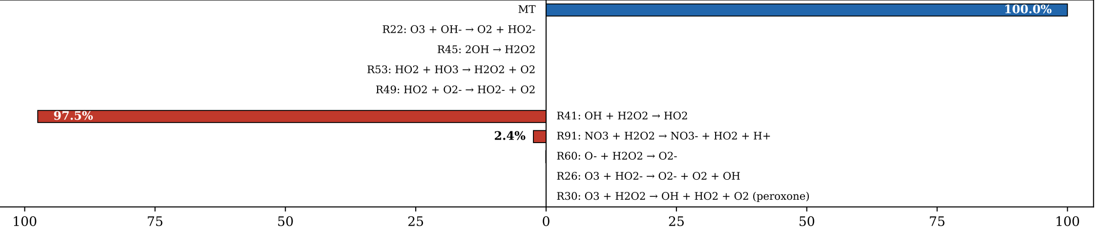
(d) H 2 O 2 (Σsrc = 2.78e-08 M/s)
